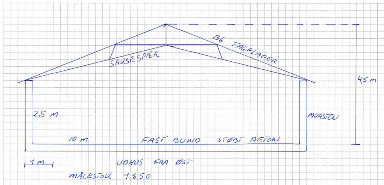
Figur 4 Ansøgers snittegning.
