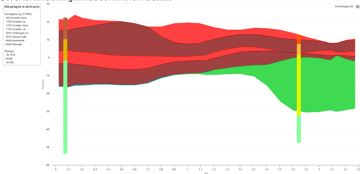
Figur 1 - Tværsnit fra boring mod øst over Faldbæk
